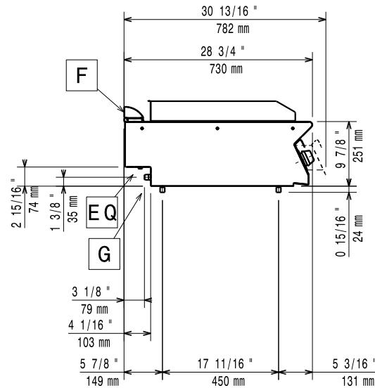
Oldalnézet
